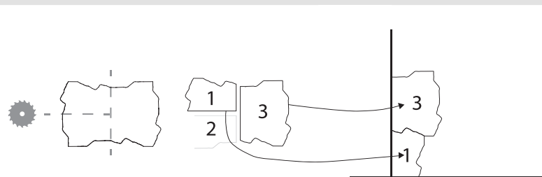
Schéma de découpe et démarrage de pose N°1
